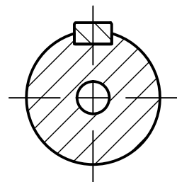
SECTION A-A SCALE 1:4
