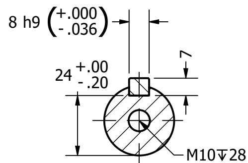
SECTION A-A SCALE 2:3
