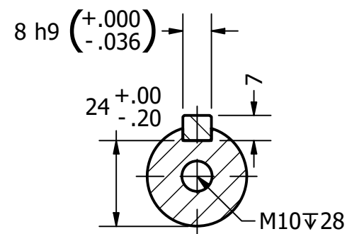
SECTION A-A SCALE 2:3
