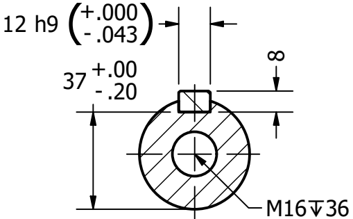
SECTION A-A SCALE 1:2
